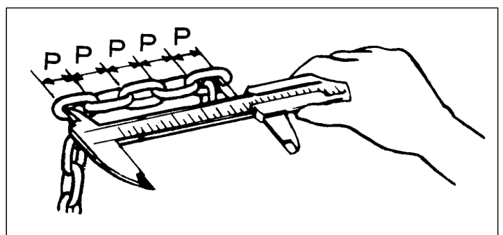
Kuva 7 Ketjun mittaus
