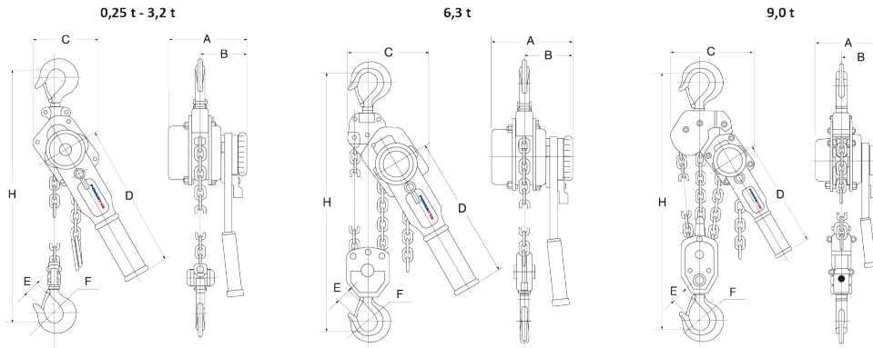
Kuva 1 Mittapiirros
