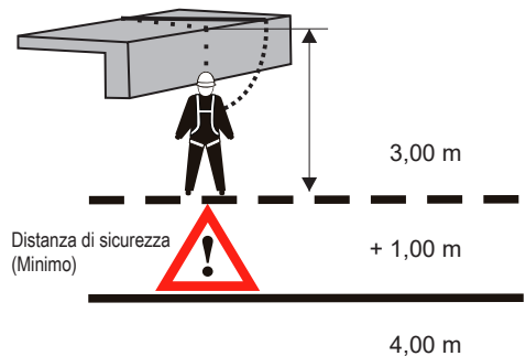
16 Caduta laterale oltre i bordi
