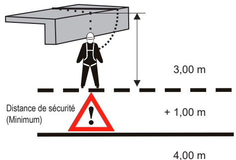
16 chute latérale par-dessus bord
