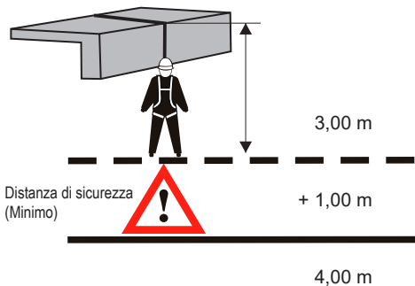
15 Caduta ad angolo retto oltre i bordi
