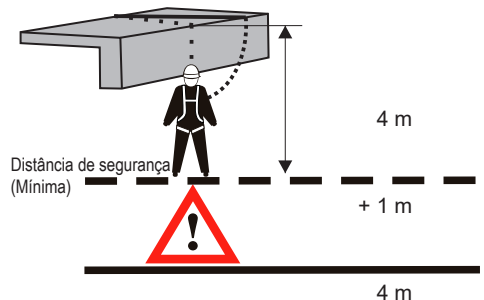
16 queda lateral sobre bordas
