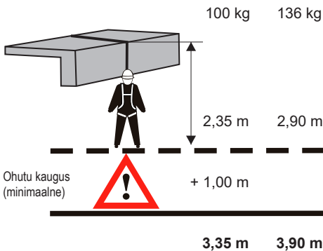
15 Kukkumine üle serva parempoolse nurga all
