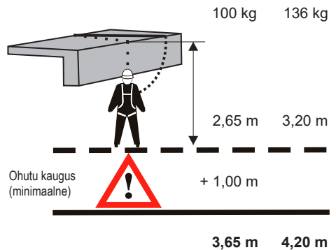
16 Kukkumine üle serva küliti
